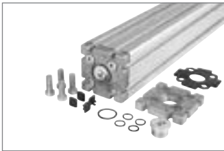
Piastra flangiata (pag. 5-3)
