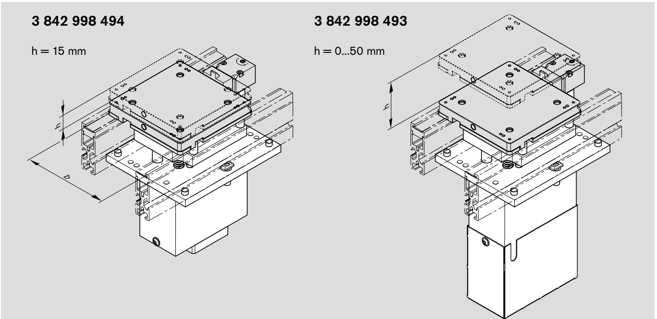
Unità di sollevamento e posizionamento HP 1/P Unidad de elevación y posicionamiento Unidade de elevação e posicionamento
