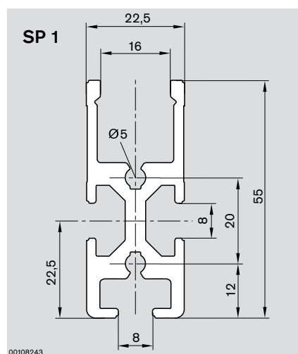
Profilato tratto SP 1 Perfil de tramo Perfil de via
