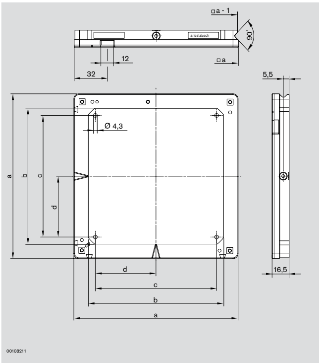
Pallet WT 1/S Portapiezas Pallet porta-peça
